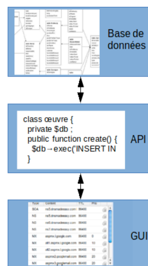
Figure 1: Architecture de la base Presto et de ses interfaces
