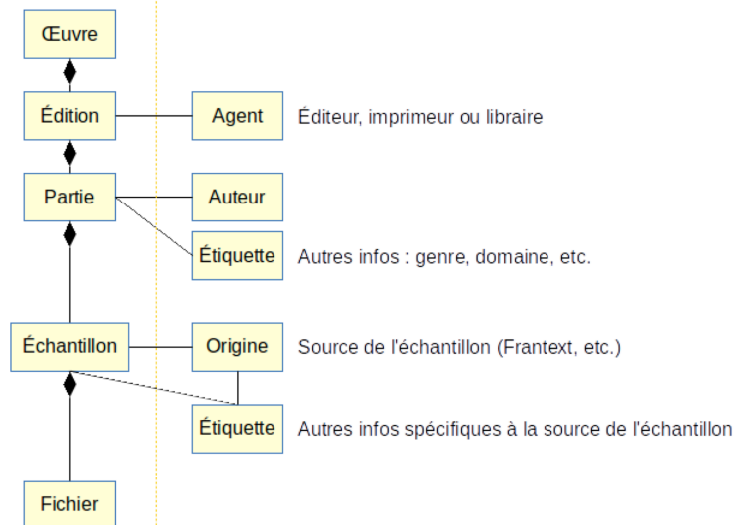
Figure 2: Structure (simplifiée) de la base de données.
